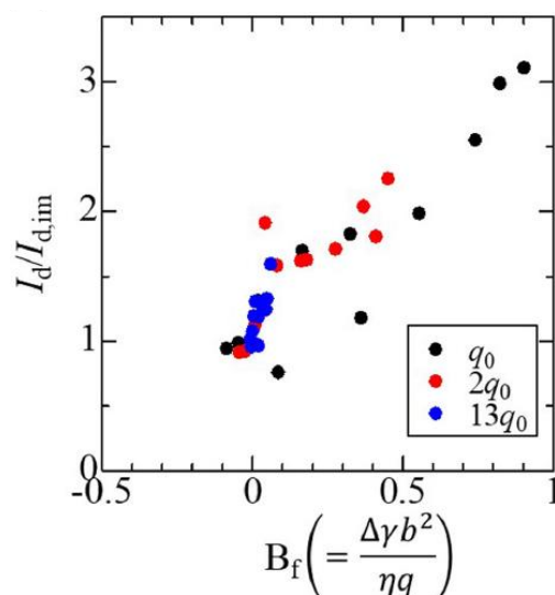
図 3 界面の変形度と無次元数 B_f の関係 縦軸は界面の変形度 I_d を非混和系の界面の変形度 I_{d,im} で規格化した値。横軸 B_f の式中、 \Delta\gamma は図 2 より求められる界面張力の経時変化量、 b はヘレ・ショウセルの間隔、 \eta は高粘性溶液の粘度、 q は注入流量。 B_f が大きくなるほど、相対的に相分離の際に生じる体積力の寄与が大きくなる。
